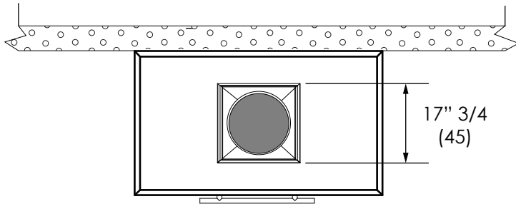
VISTA PLANTA
