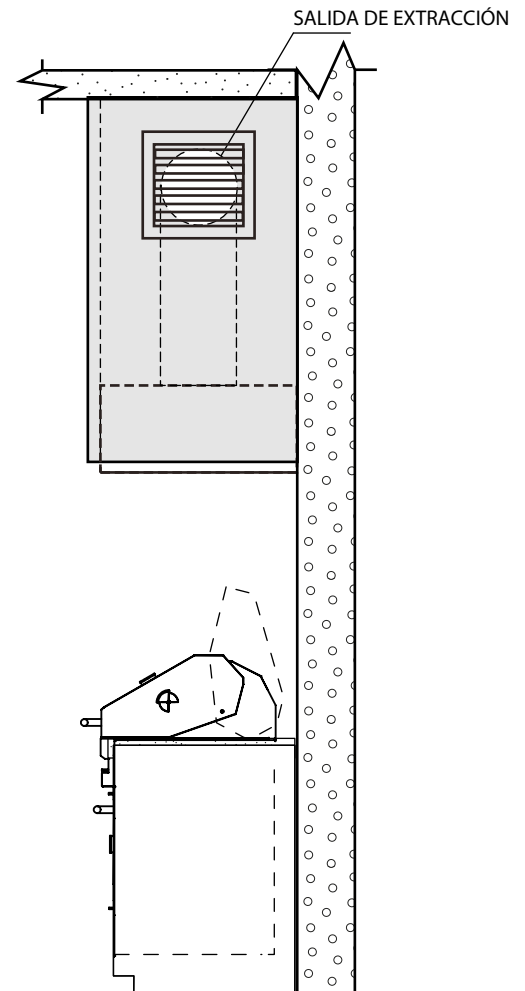
VISTA LATERAL
